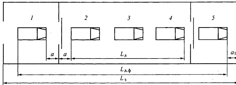
Рис. 2.3. Схема планировки поточной линии с тамбурами:
