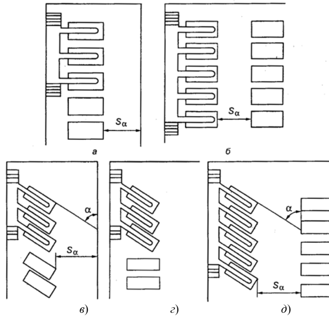
Рис. 3.2. Варианты расположения постов в производственных помещениях:
