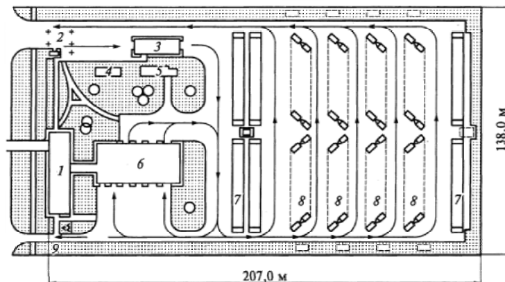
Рис. 4.1. Схема генплана АТП на 200 грузовых автомобилей при моноблочном строительстве с отдельно стоящей линией мойки:
