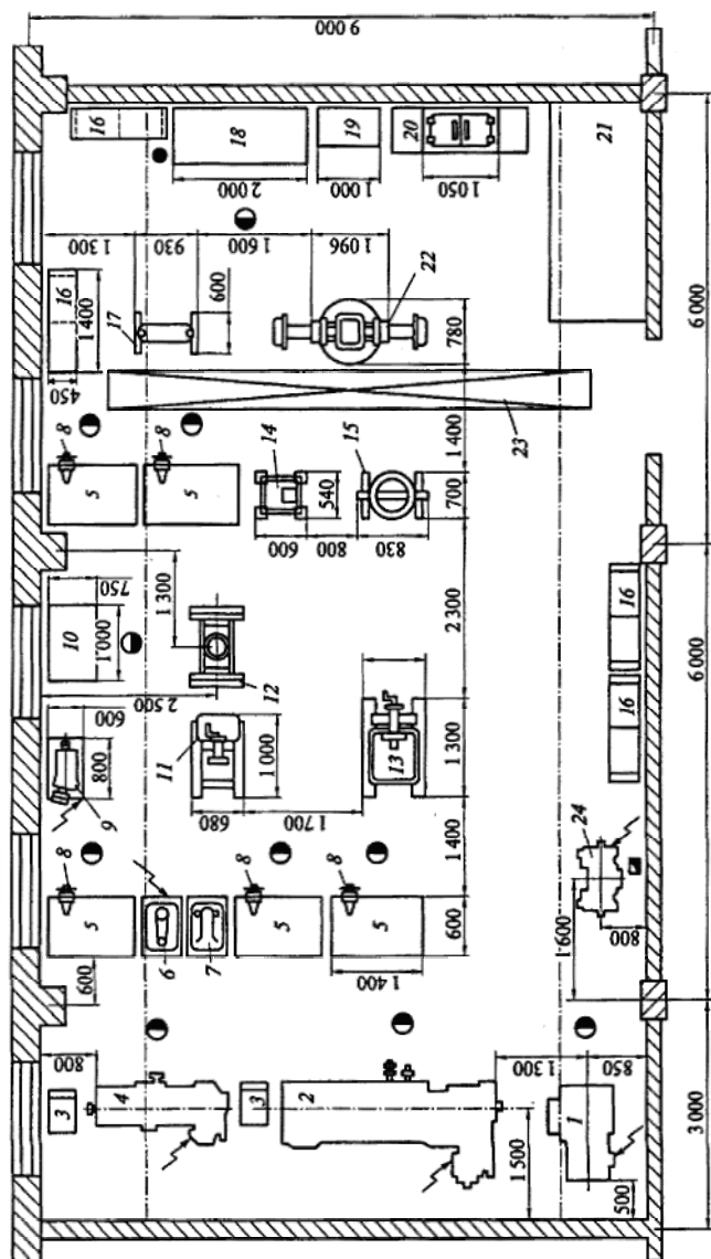
Рис. ПЗ. Планировка агрегатно-механического цеха АТЦ:
