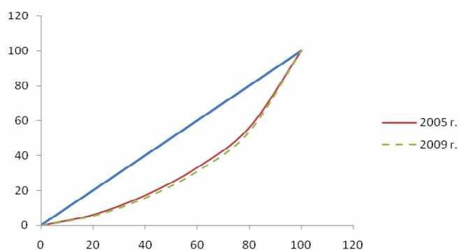
Рис. 4. Кривая Лоренца
