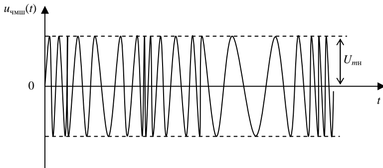
Рис. 2.19. Осциллограмма ЧМШ помехи
