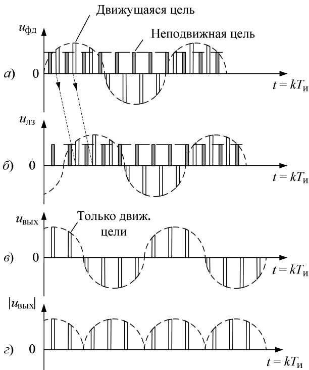
Рис. 3.18. Принцип работы схемы ЧПК
