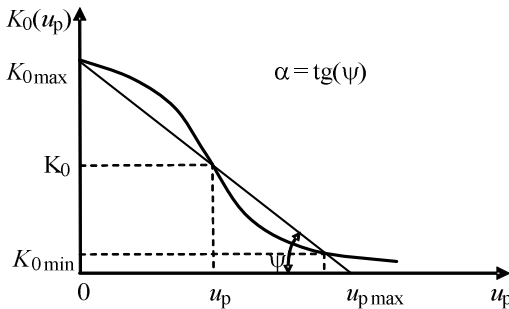
Рис. 3.6. Зависимость K_0(u_p) от u_p
