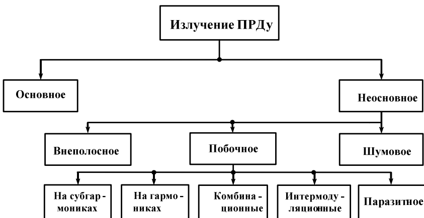
Рис. 4.2. Классификация излучений передающего устройства
