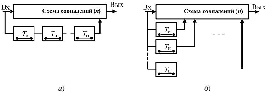
Рис. 3.22. Схемы селекции импульсов по частоте повторения
