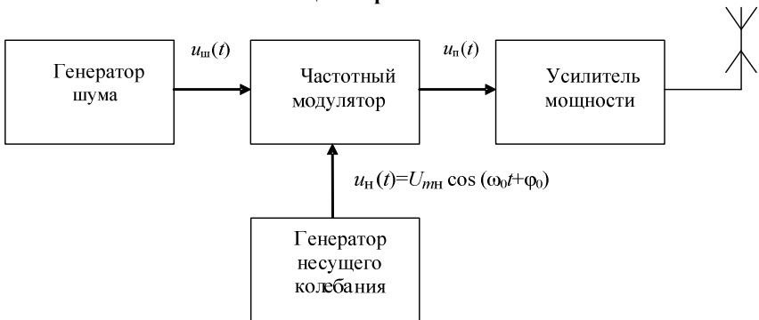
Рис. 2.20. Схема формирования ЧМШ помехи
