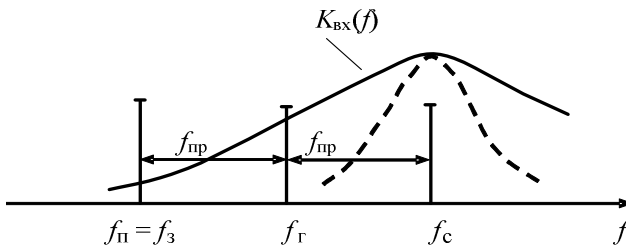
Рис. 4.6. Образование зеркального канала приёма при нижней настройке гетеродина
