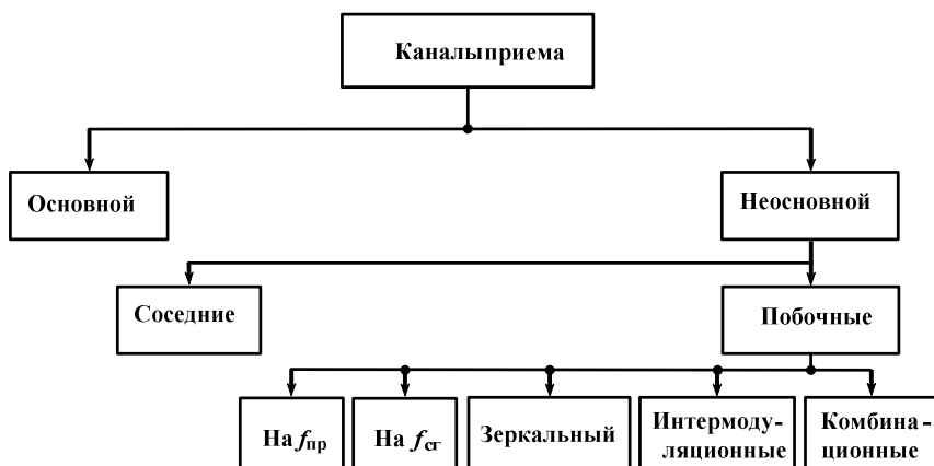
Рис. 4.3. Классификация каналов приёма радиосигналов
