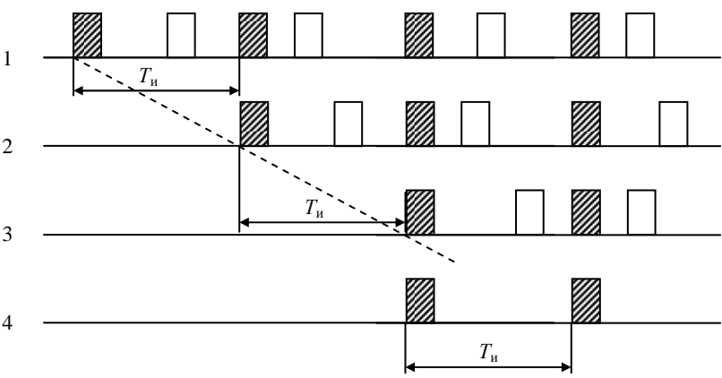
Рис. 3.23. Диаграмма работы схемы для 3-импульсной схемы совпадений
