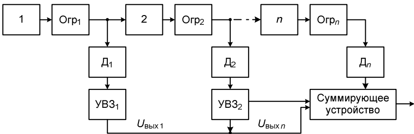
Рис. 3.3. Функциональная схема ЛУ с последовательным включением каскадов
