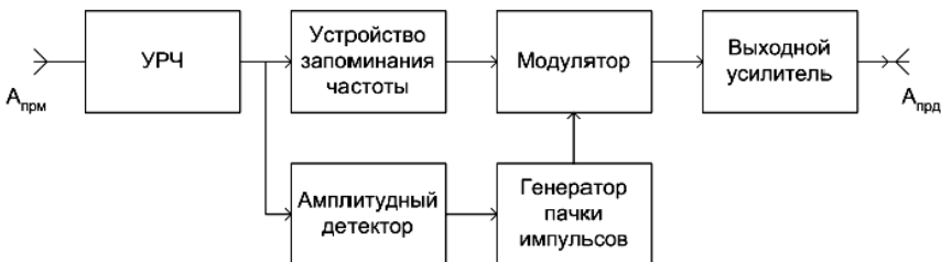
Рис. 2.27. Структурная схема передатчика МПП
