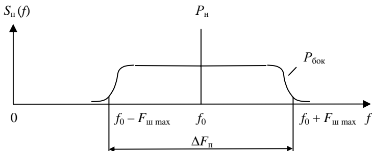
Рис. 2.22. Спектральная плотность боковых составляющих и мощность несущего колебания ЧМШП
