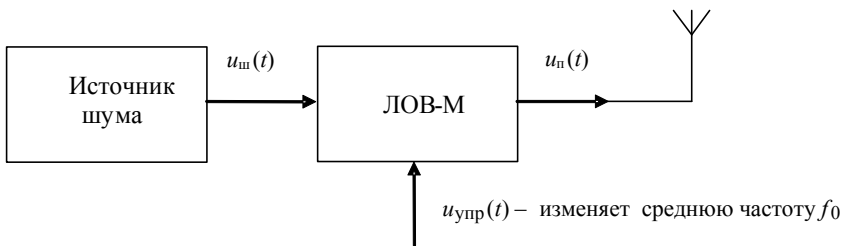
Рис. 2.21. Схема формирования ЧМШ помехи на ЛОВ-М
