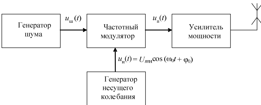
Рис. 2.18. Схема формирования ЧМШ помехи
