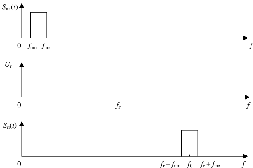
Рис. 2.16. Спектральные диаграммы, поясняющие формирование ППП сигнала методом гетеродинирования
