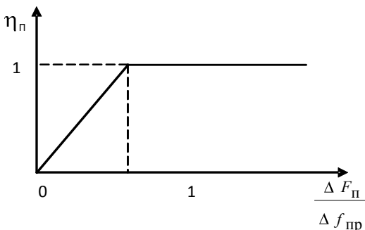
Рис. 2.12. Зависимость коэффициента качества помехи от ширины спектра помехи
