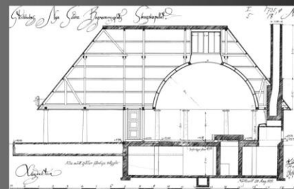
Лесная часовня, продольный разрез
