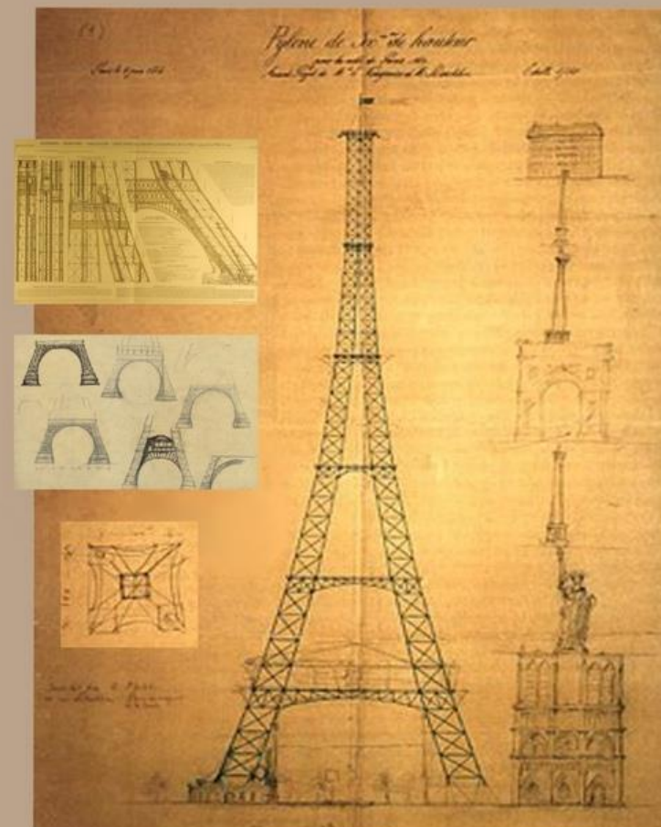
Эйфелева башня
