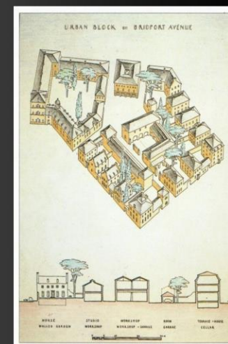
«Городской квартал на Бридпорт-авеню»
