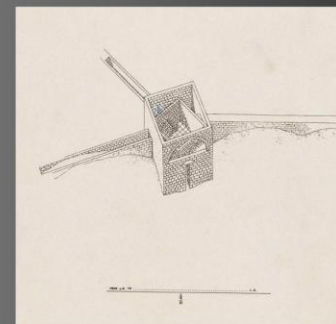
«Дом Колина Роу», 1975 Аксометрический вид с воздуха. Бумага, тушь, гуашь
