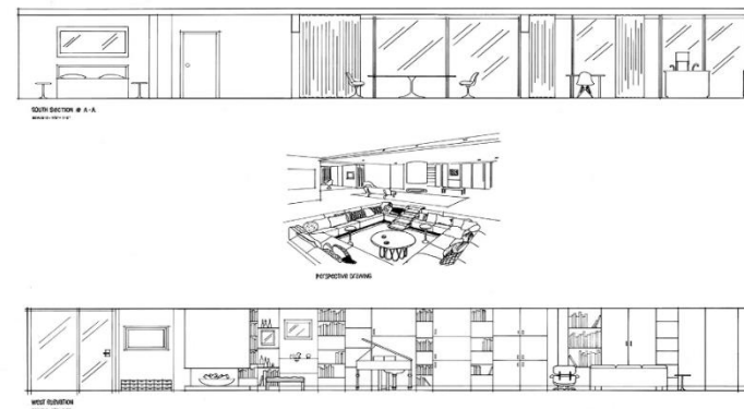
Эскиз интерьера дома Миллера
