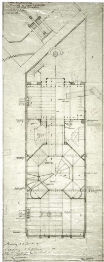
План первого этажа особняка Этвельде, 1897 г.
