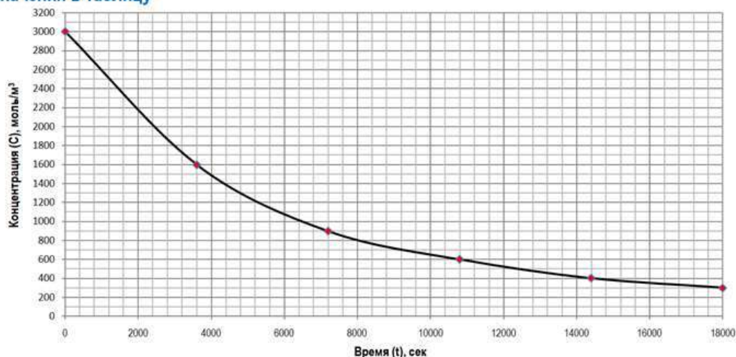
Кинетическая кривая истощения надпероксида калия хемосорбентом
