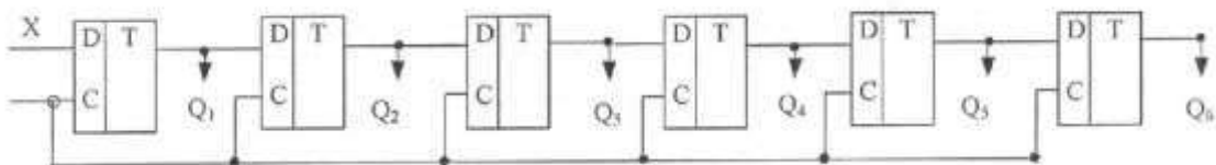
Рис. 5. Схема последовательного шестirazрядного регистра
