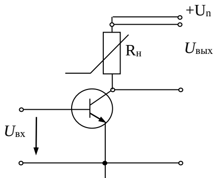
Рис. 3. Источник тока на биполярном транзисторе
