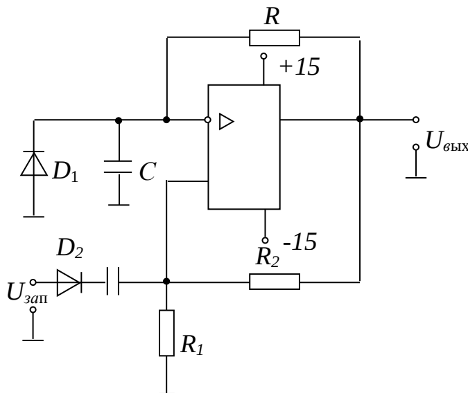
Рис.2. Схема одновибратора
