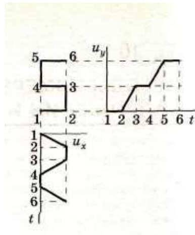
Рисунок 7 – Функции u_y(t) и u_x(t) для получения на экране цифры 5 по шрифту Бергера
