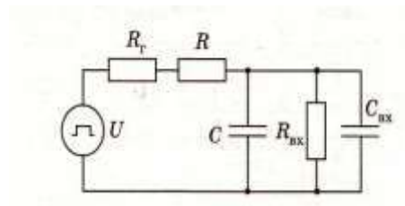
Рисунок 5 – Эквивалентная схема измерения u_c(t)
