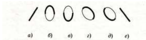
Рисунок 8 – Измерение знака сдвига по фазе
