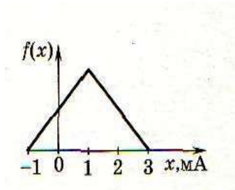
Рисунок 1 – Треугольное распределение
