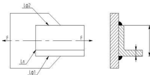
Рис. 4. Уголок, приваренный к косынке
