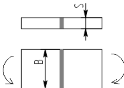
Рис. 3. Действие момента на стыковое соединение
