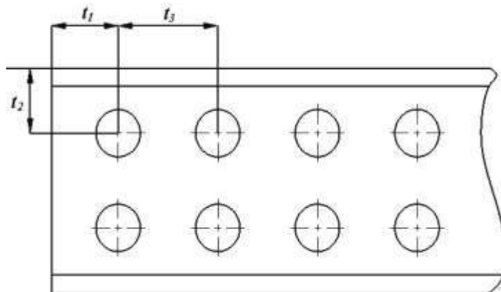
Рис. 6. Расстановка сварочных точек
